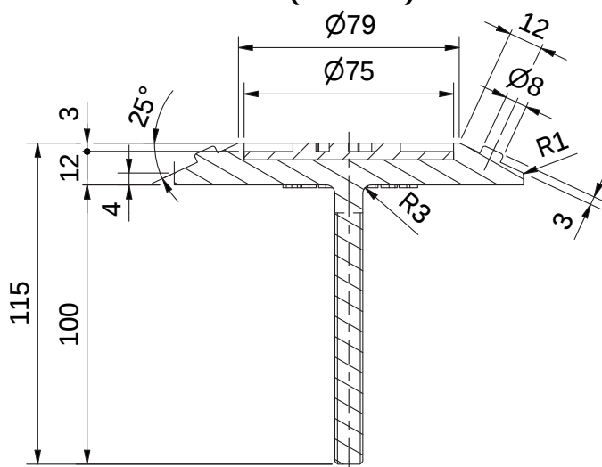
SECTION A-A ( 1 : 2 )
